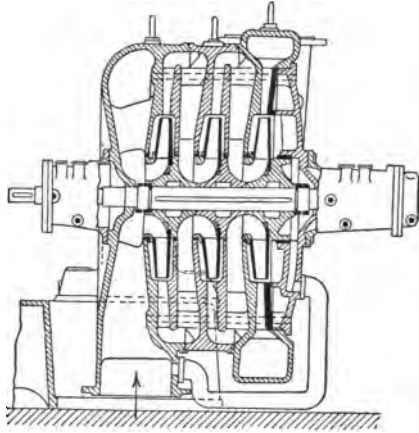
FIG. 95.—Jaeger's turbo-blower.
